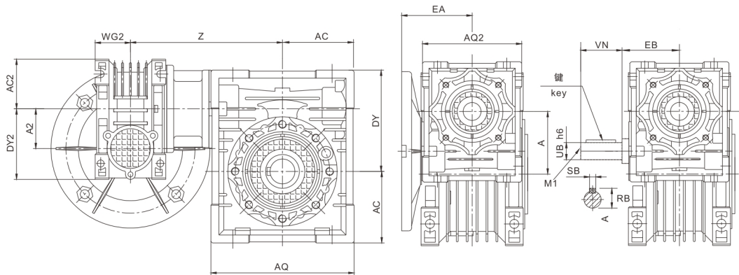
JRSTE(D)安装尺寸 JRSTE( D) Mounting Dimensions
