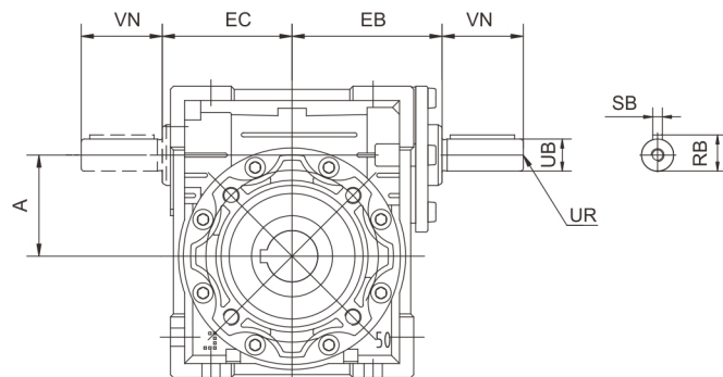
JRWN(B) 英制产品安装尺寸 JRWN(B) Mounting Dimensions
