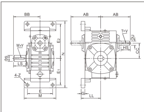
WPV 轴指向表示 SHAFT DIRECTION
