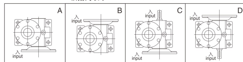
轴指向表示 SHAFT DIRECTION
