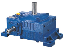
WPWO 轴指向表示 SHAFT DIRECTION
