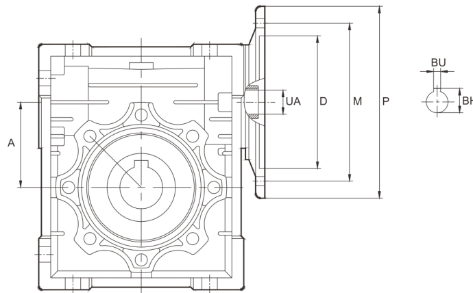
NEMA电机输入法兰 NEMA Motor Input Flange
