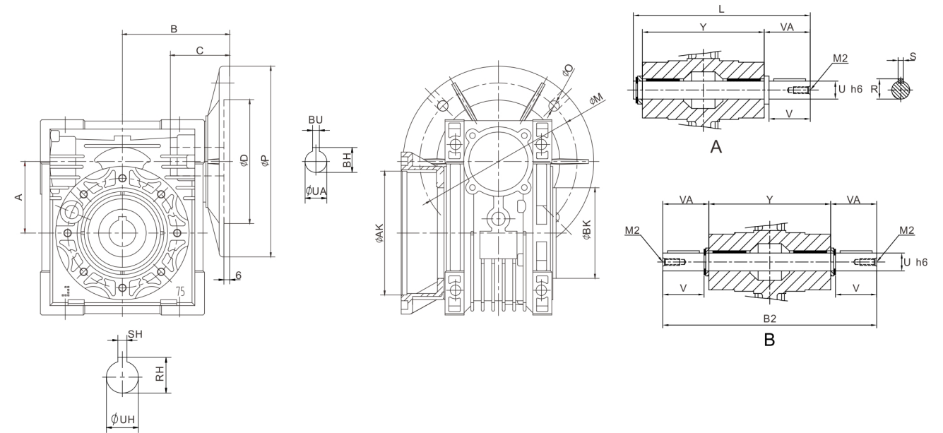
JRWND英制产品重要接口尺寸表 JRWND Important Connect Size
